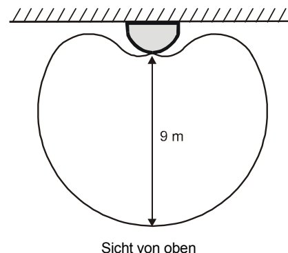
Erfassungsbereich des Glasbruchsensoren
